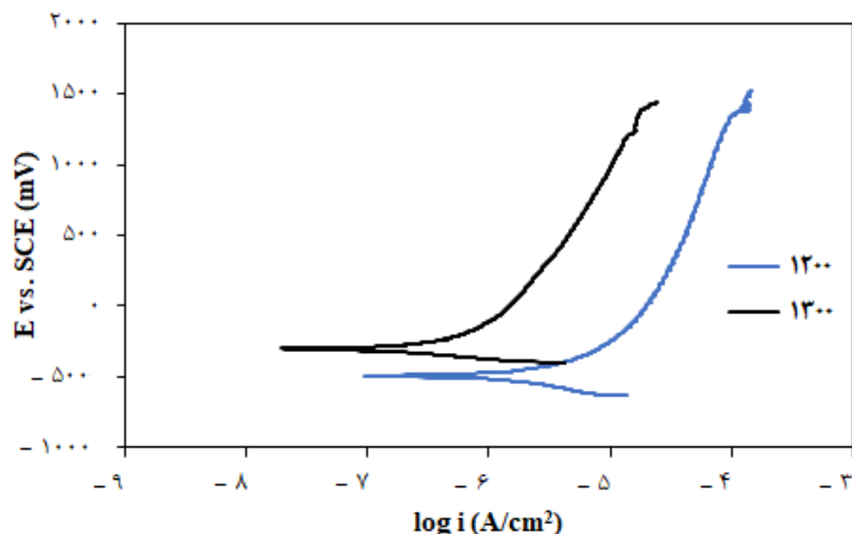
شکل ۸- منحنی‌های پلاریزاسیون نمونه‌ها در محلول رینگر.
